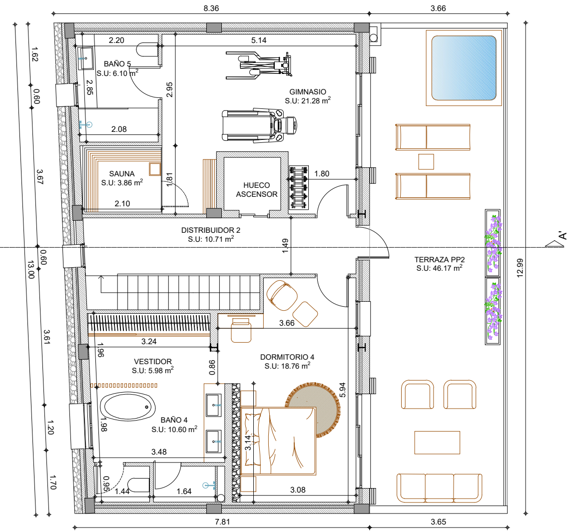
PLANTA PISO 2 SECOND FLOOR ERSTES OBERGESCHOSS
